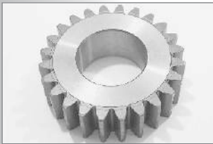
Ford-Eixo Engrenagem Cod. Orig. 5125328 Cod. Enfer 1008529
