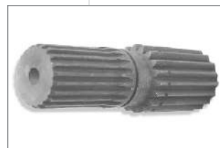
ZF-Eixo Solar Cod. Orig. 4472352074 Cod. Enfer 1001125
